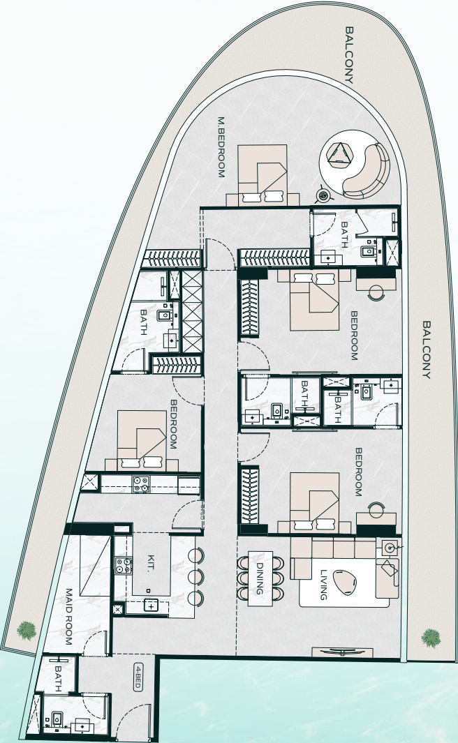
4 BEDROOM TYPE 01
